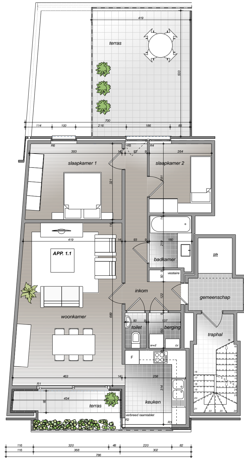
GRONDPLAN 1-100
